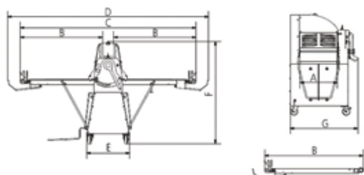
ST500-50/70/85/100/120
