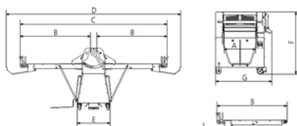
SF600-85/100/120/140
